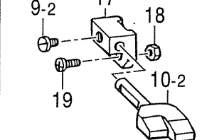
< 移動針受用 >
