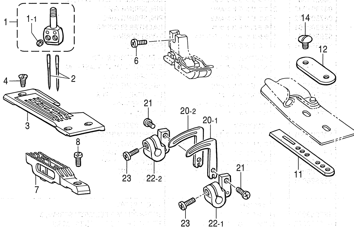
< -2 3/16 固定針受用 >
