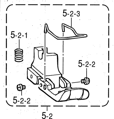
< 1/8, 5/32 用 >
