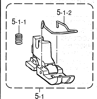
< 固定針受用 >
